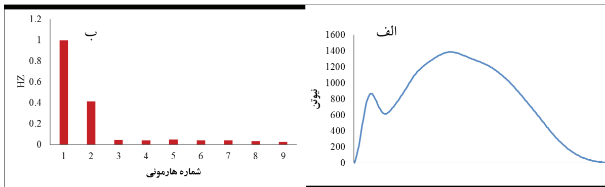
شکل ۱: تبدیل فوریر GRF در تابع زمان (ب) طیف توان GRF
